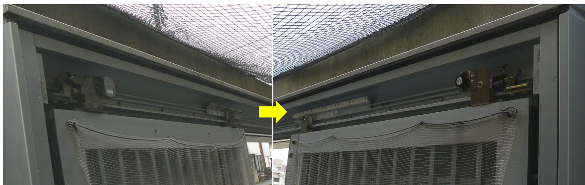
引戸クローザ修理 (5月14日) 部品交換、制動ラック2個→3個
