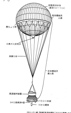
風船爆弾全体図→
