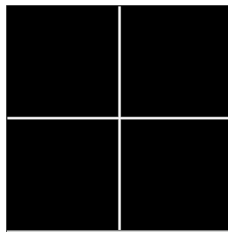
図 2.5: Steiner のローマ曲面, Z=0
