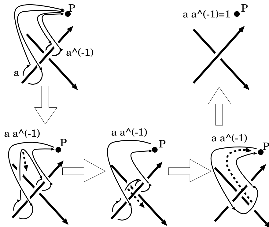
図 1.8: 閉じた道 a , a^{-1} と aa^{-1} の意味
