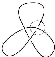
図 1.14: クローバー結び目
