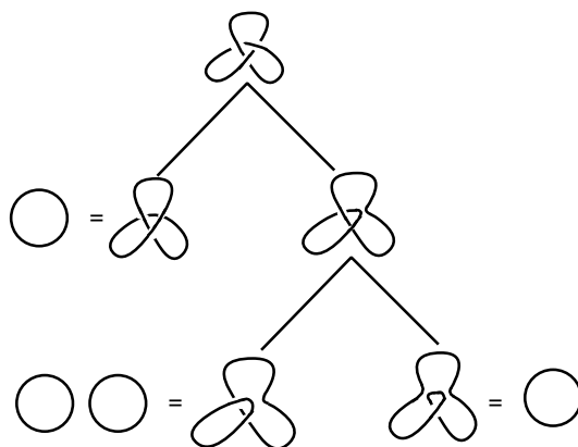
図 1.15: クローバー結び目のスケイン関係
