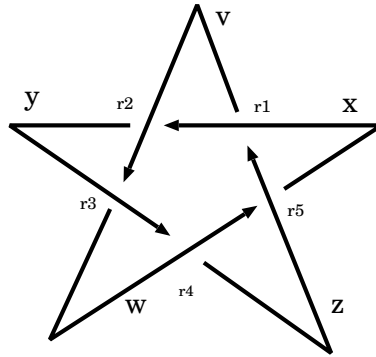
図 1.5: 星型結び目 5_1 と変数
