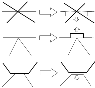
図 1.3: 変形可能な交点
