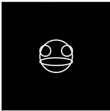
図 2.2: アヒル?
