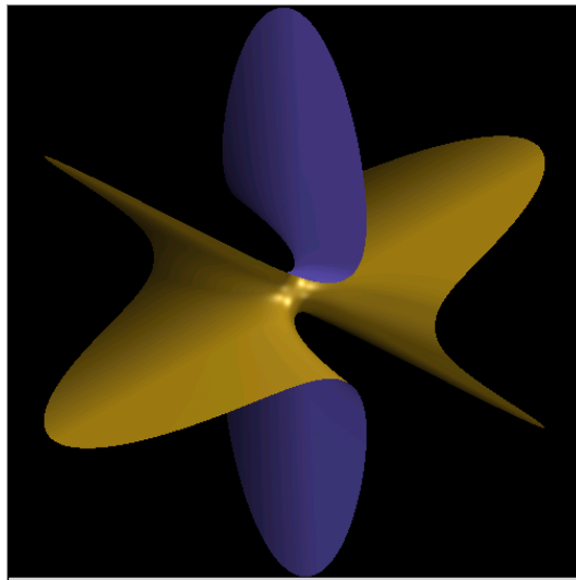
図 2.6: 猿の腰掛
