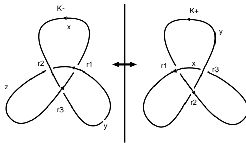
図 1.13: クローバ結び目の鏡像
