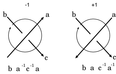
図 1.6: Wirtinger 表示
