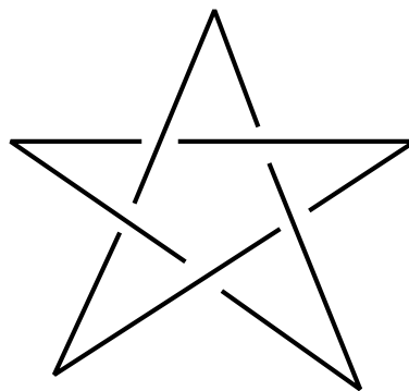
図 1.1: 星型結び目 ( 5_1 )
