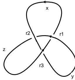
図 1.10: クローバー結び目 ( 3_1 )
