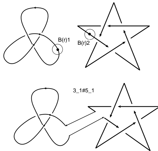
図 1.11: 結び目 3_1 と 5_1 との連結和
