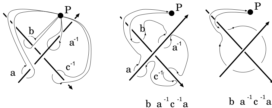
図 1.9: Wirtinger 表記の意味
