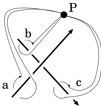
図 1.7: 結び目と閉じた道
