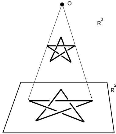
図 1.2: 結び目の射影図
