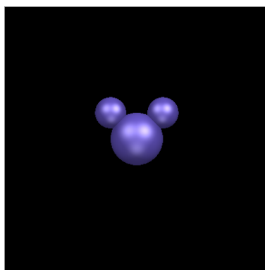
図 2.1: ? 曲面
