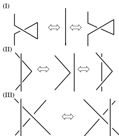
図 1.4: Reidemeister 変形
