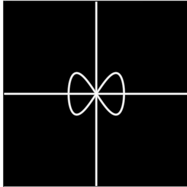
図 2.3: レムニスケート
