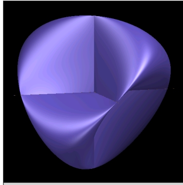
図 2.4: Steiner のローマ曲面
