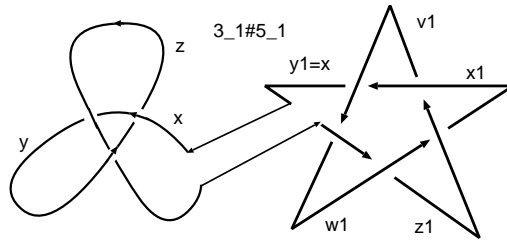
図 1.12: 結び目 3_1 と 5_1 との連結和の結び目群
